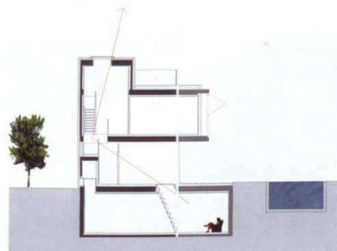
12 · SECCION TRANSVERSAL
