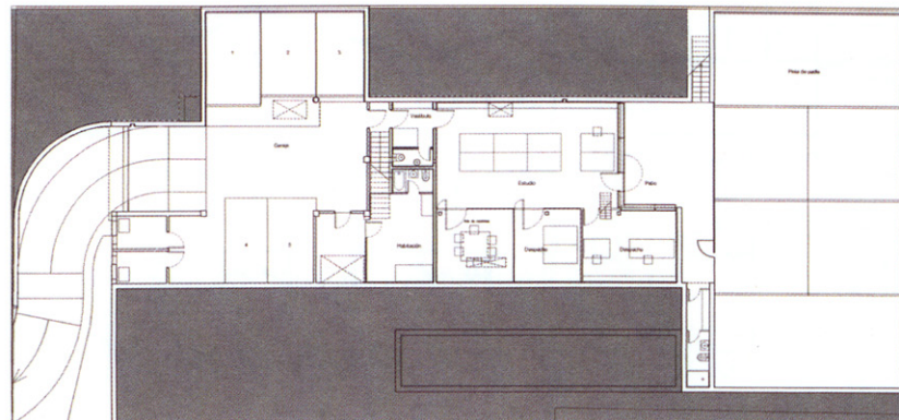
17 · PLANTA SOTANO
